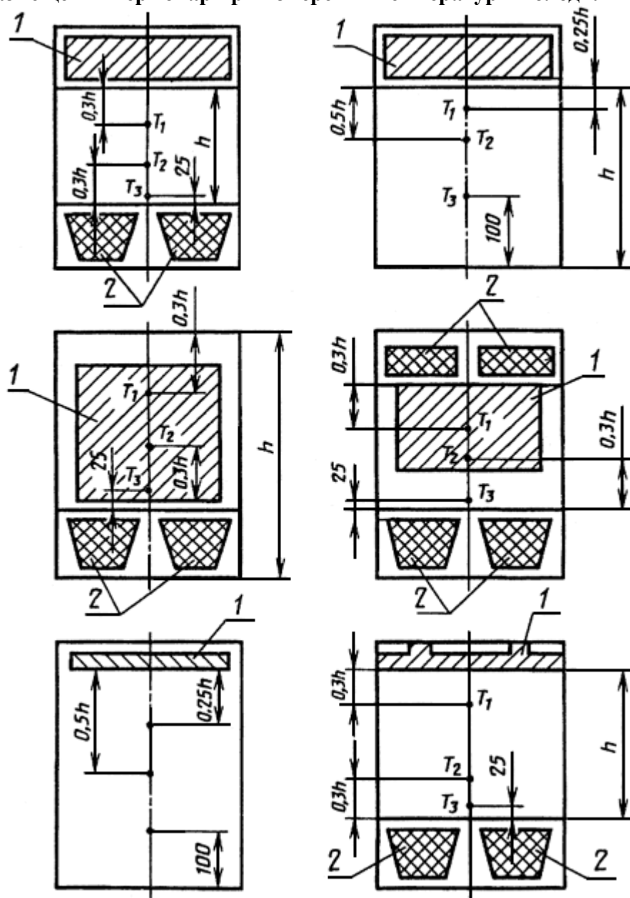
1 - испаритель; 2 - сосуд для хранения овощей; T_1, T_2, T_3 - точки измерения температур
